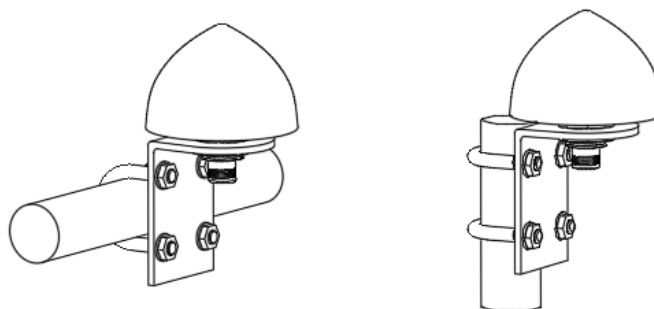
Рисунок 3.3 Крепление антенны
