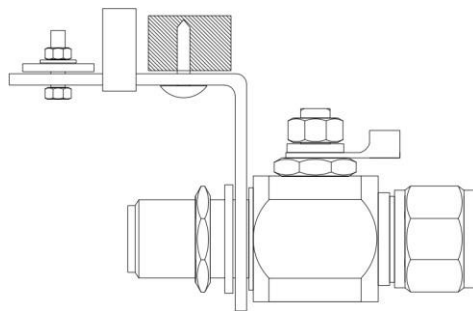
Рисунок 3.2 Крепление грозозащитника
