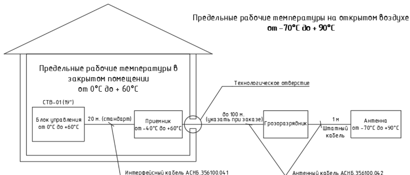
Рисунок 1.1 Подключение СТВ-01(19'') в различных температурных диапазонах.
