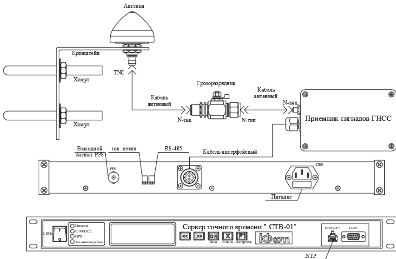
Рисунок 3.1 Схема соединения узлов СТВ-01 (19").
